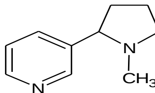
Nicotine
