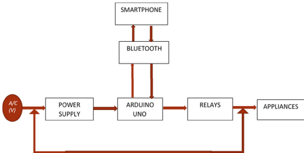
Figure3: theblockdiagramofahomeautomationsystem.
