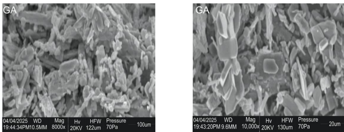
Fig 2: SEM analysis
