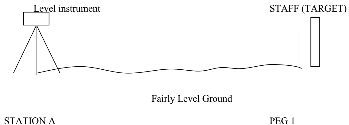
Fig3.4.1.1.: Horizontal Collimation error test
