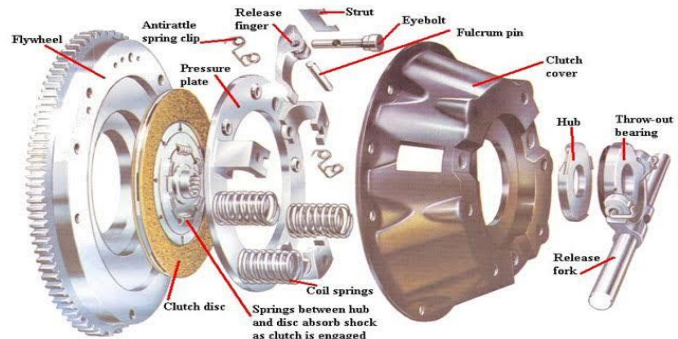
Fig. 10.1: Clutch
